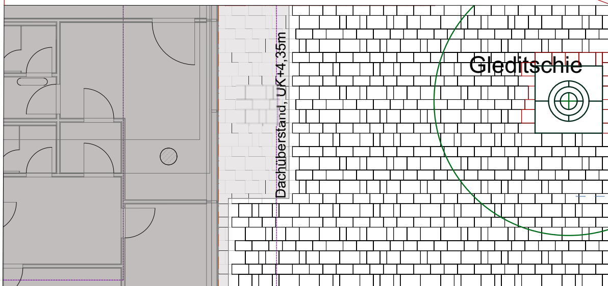
Verlegemuster M 1:100
