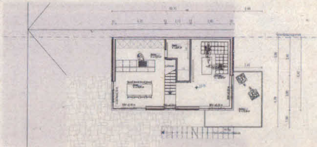
Grundriss OG
