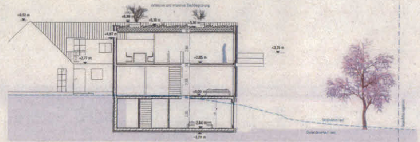
Schnitt AA
