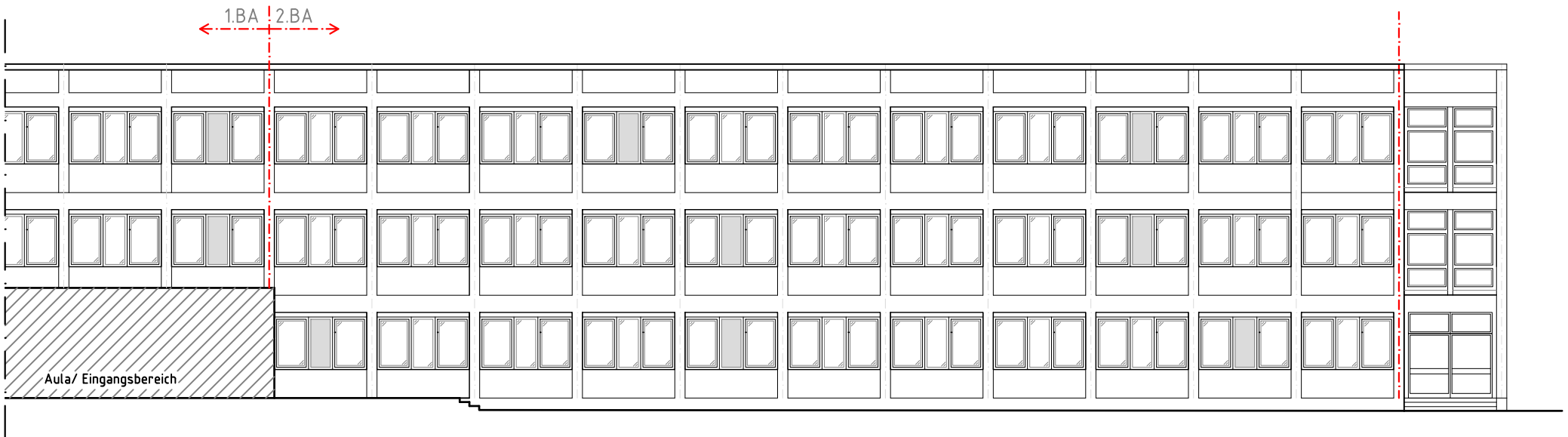
Klassentrakt Ansicht von SÜDEN
