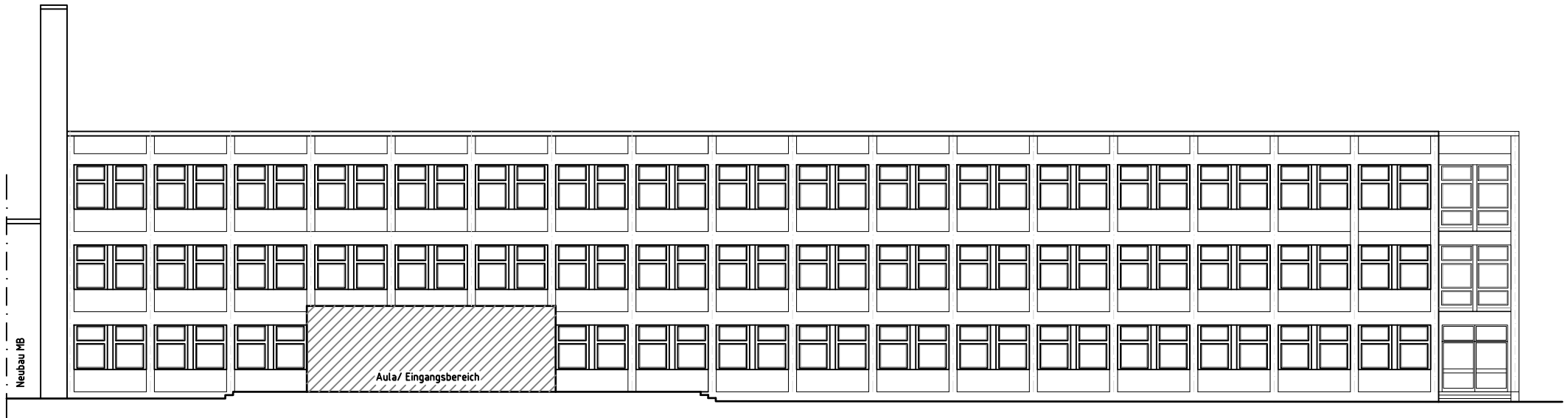
Klassentrakt Ansicht von SÜDEN Fenster BESTAND
