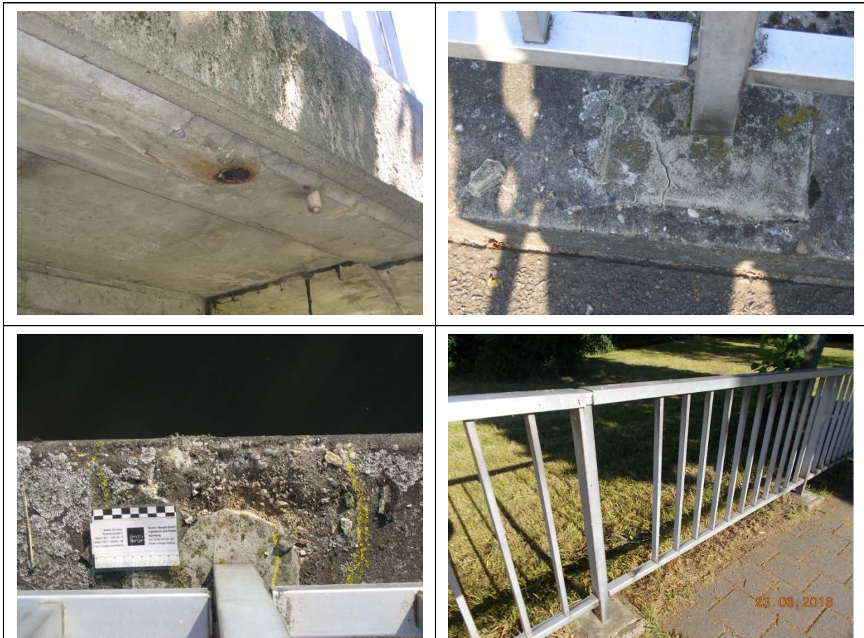
Schaden an den Gesimsen und schadhaftes Geländer
