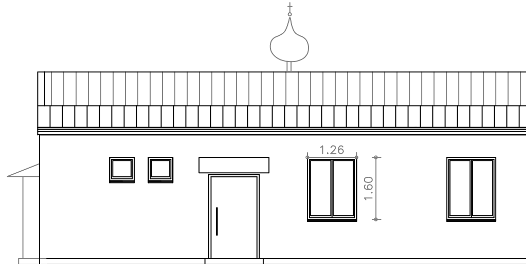
Westansicht
