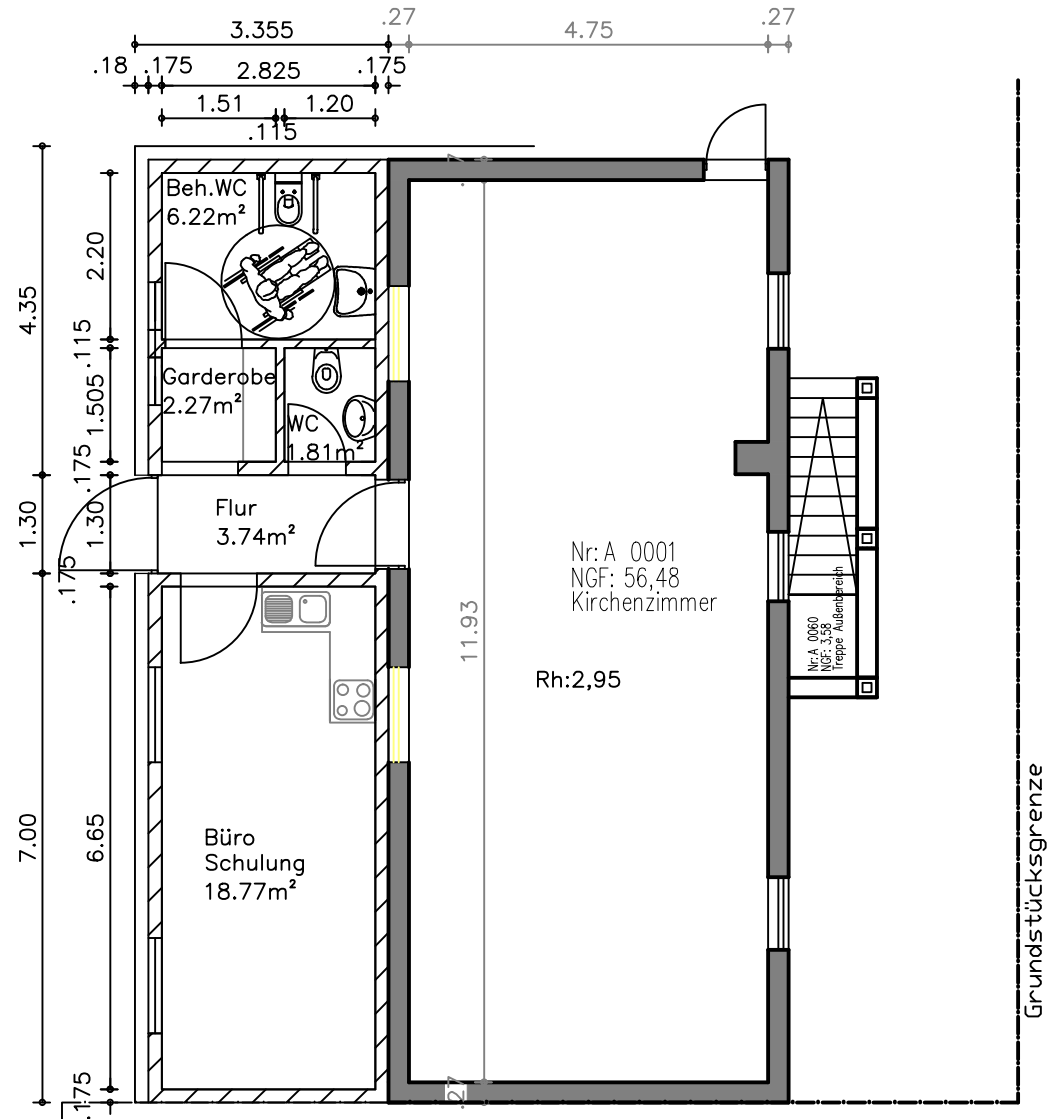
Grundriss EG
