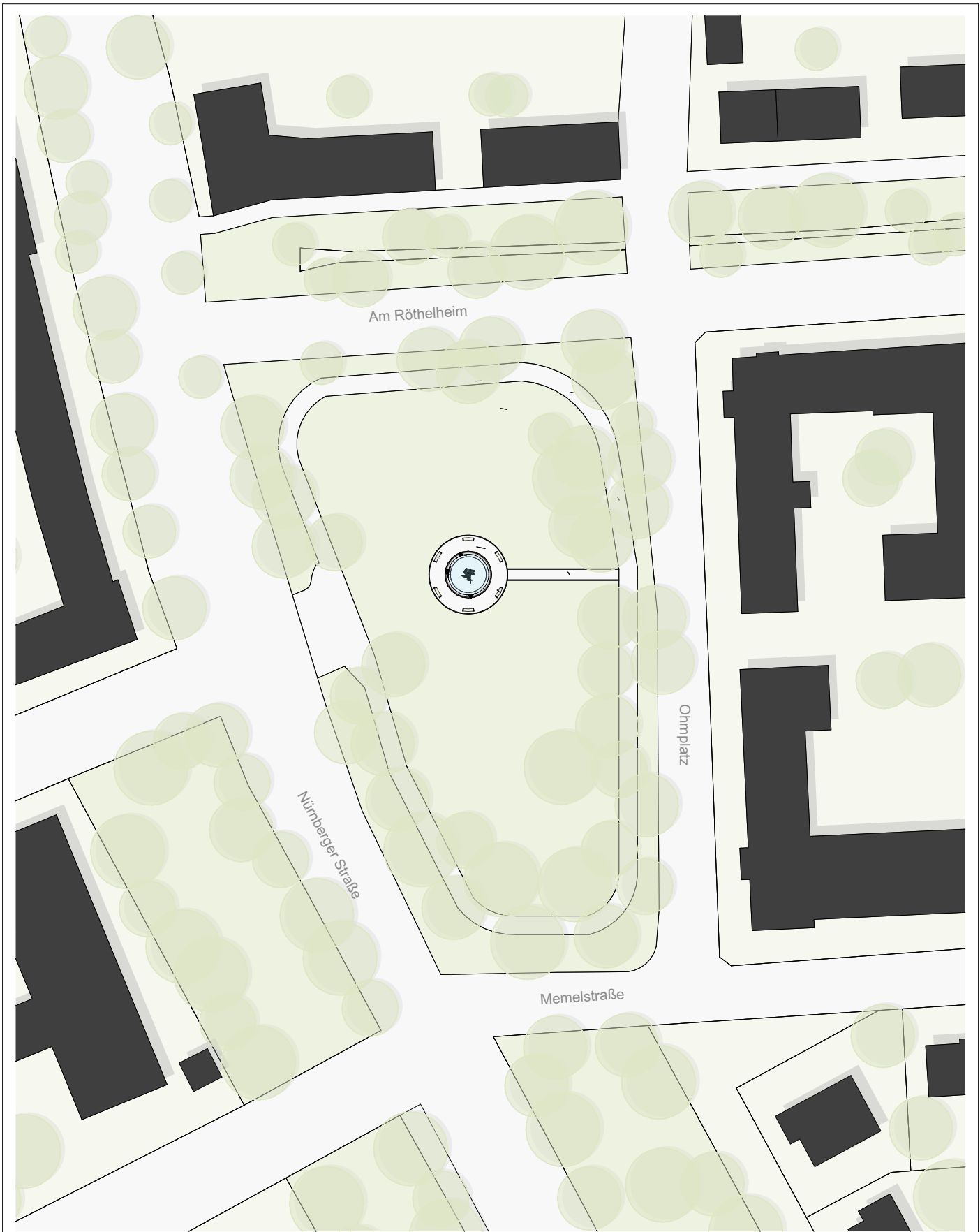
Variante 3 - Lageplan
