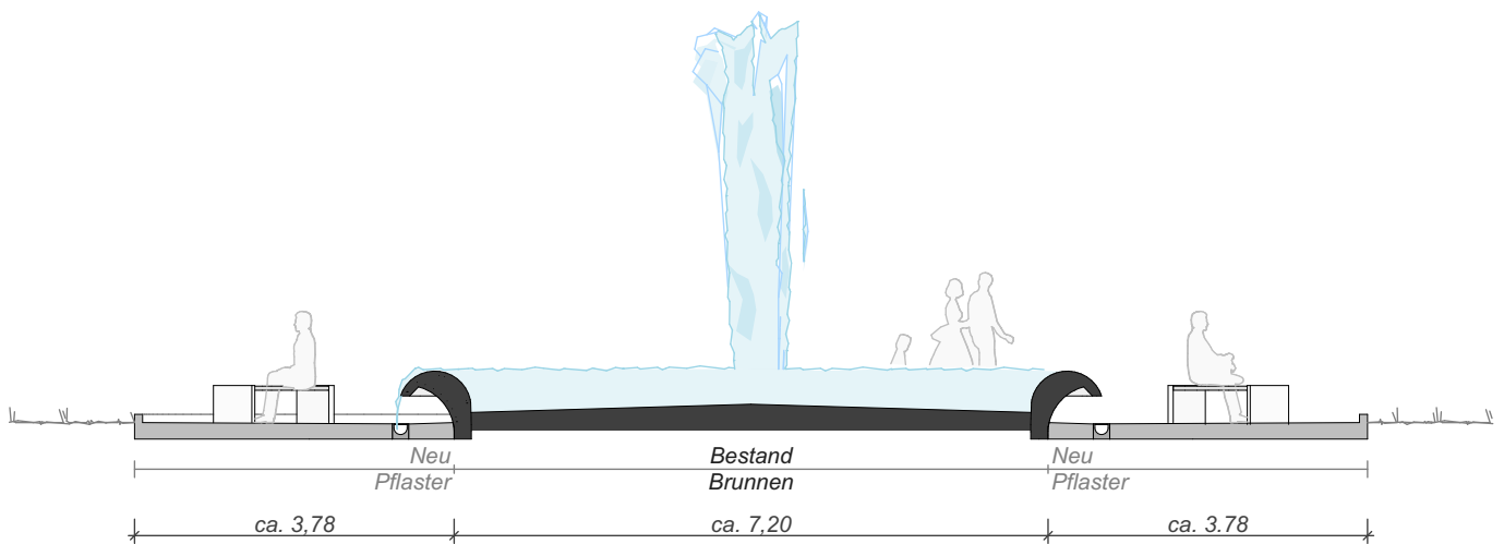
Variante 3 - Querschnitt
