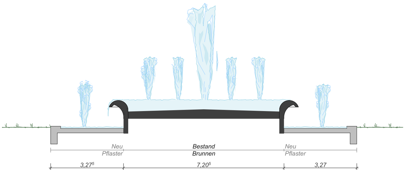
Variante 2 - Querschnitt
