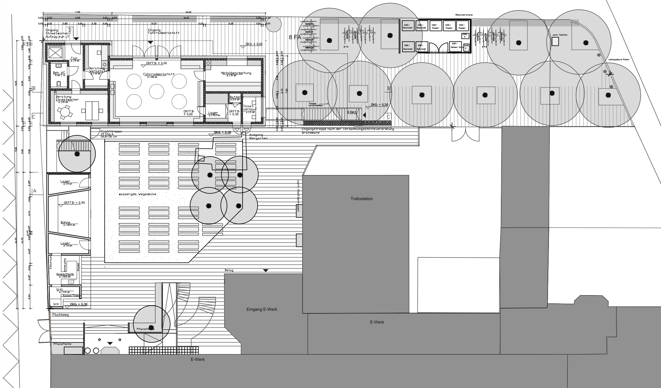
Grundriss EG
