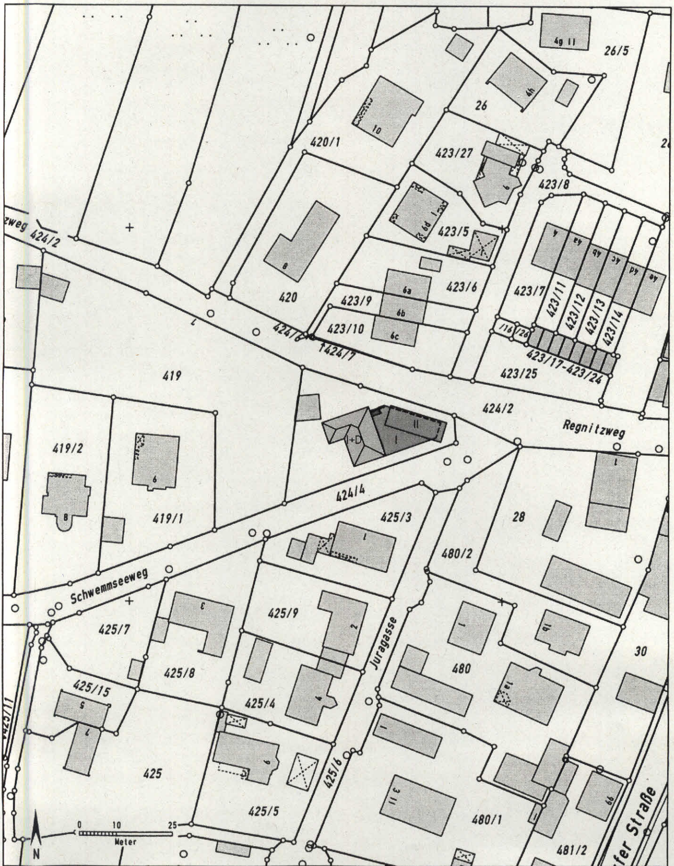
LAGEPLAN 1:1000
