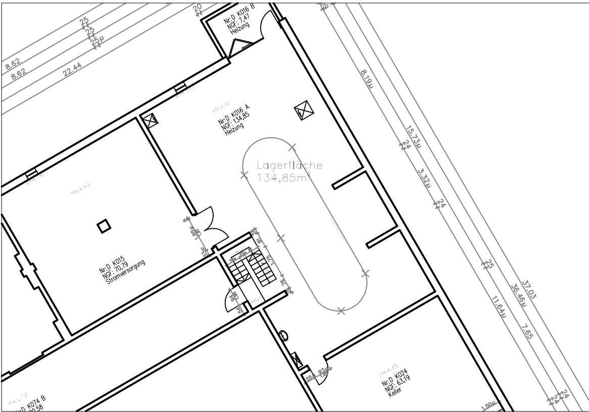
KG Grundrissausschnitt 1:200
