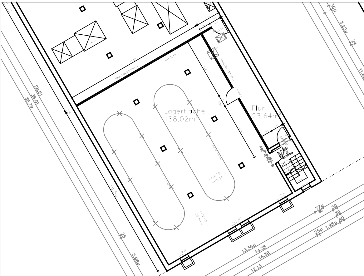
KG Grundrissausschnitt 1:200
