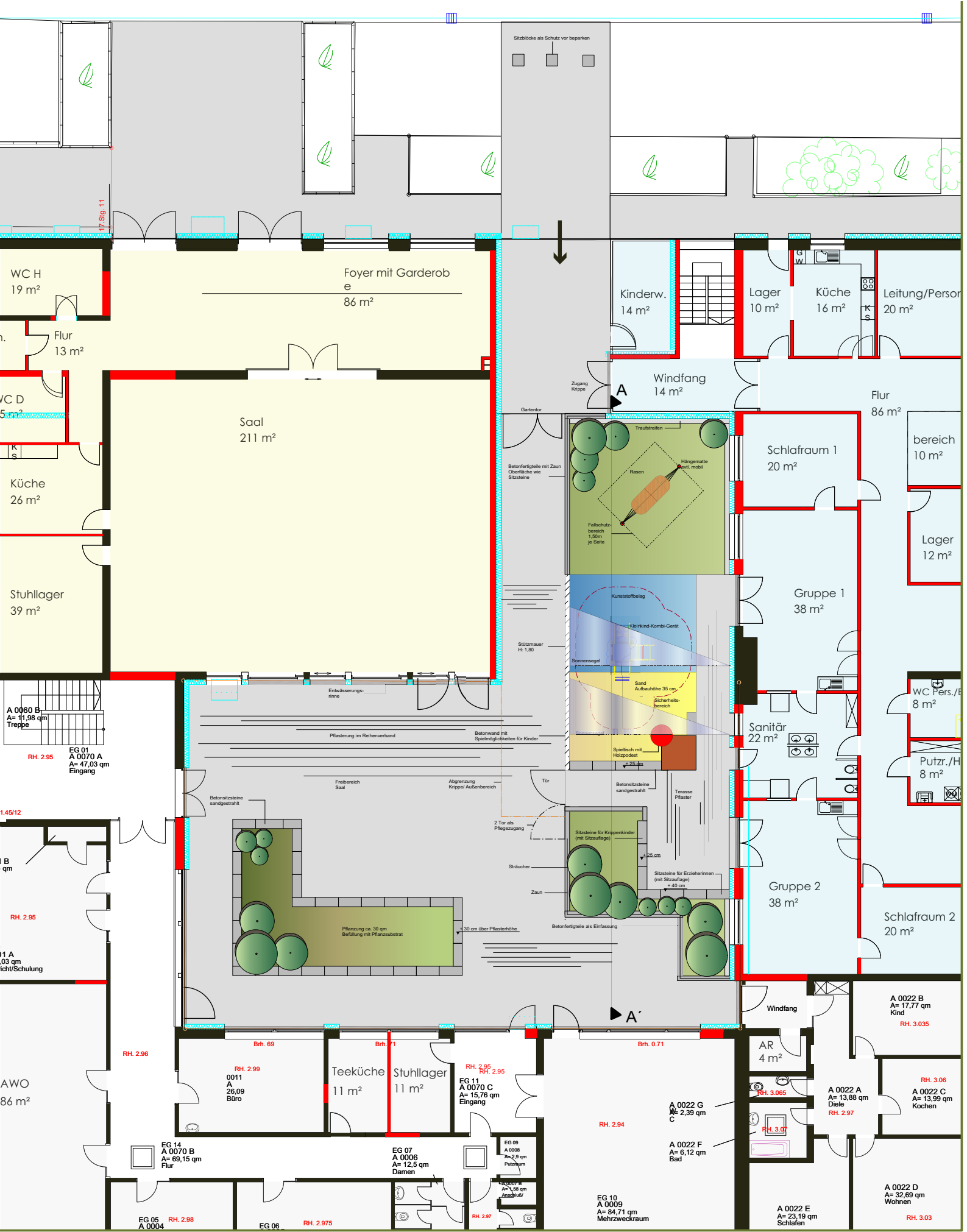
Gemeindeforum Frauenaurach - Innenhof mit Freibereich Krippe - M 1:200
