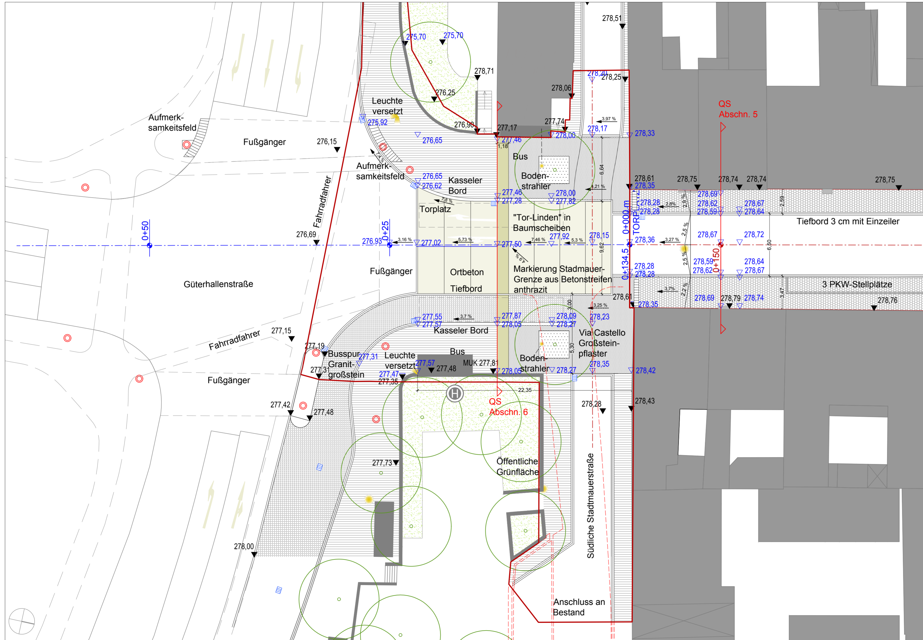
DETAL TORPLATZ
