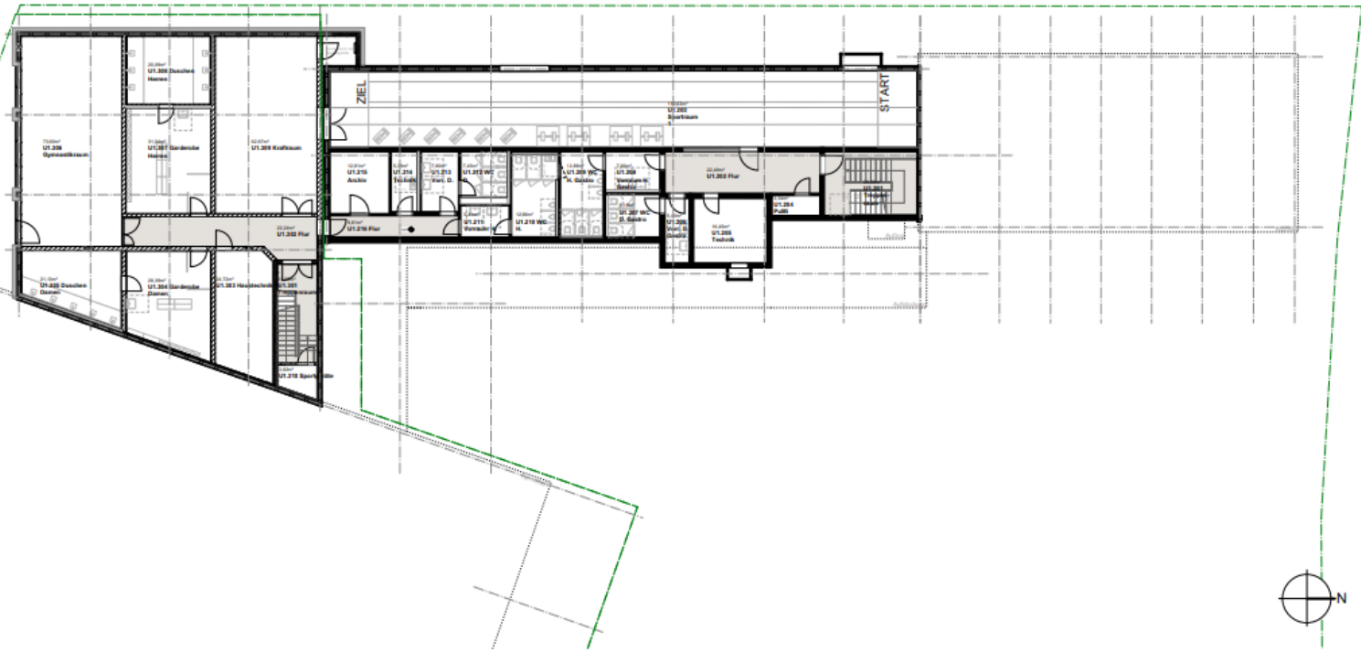
Grundriss Untergeschoss
