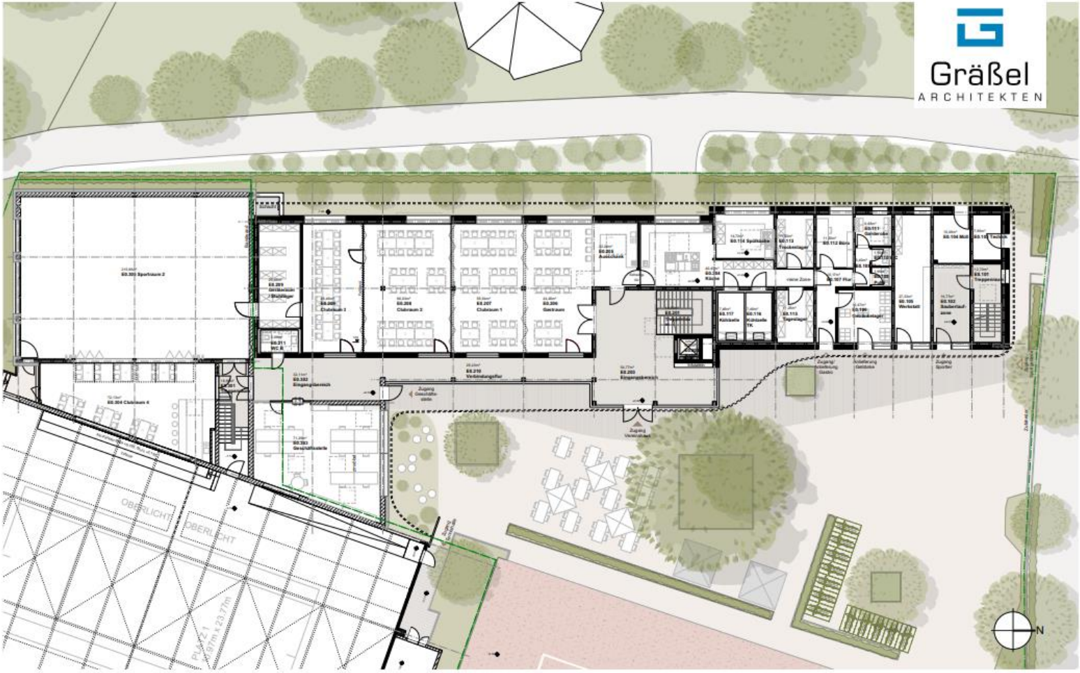
Grundriss Erdgeschoss
