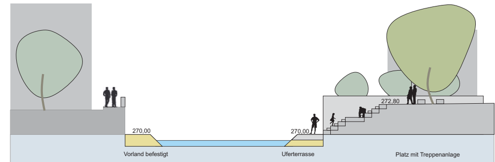
Schnitt M 1:250, verkleinert
