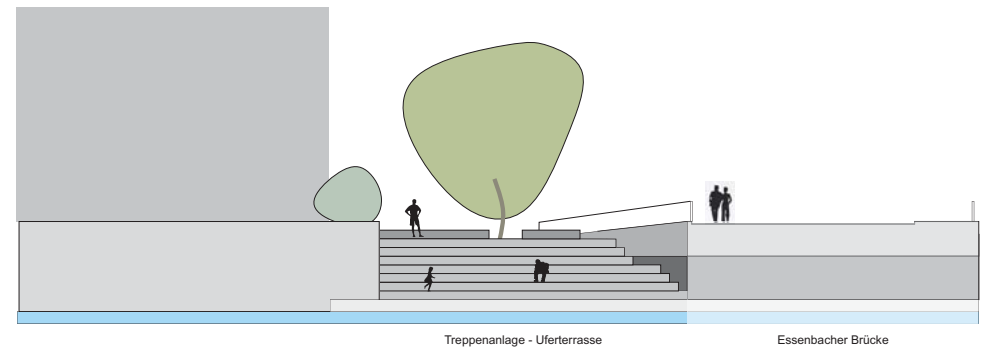
Ansicht M 1:250, verkleinert
