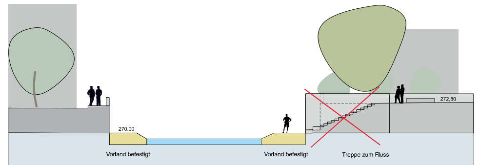
Schnitt M 1:250
