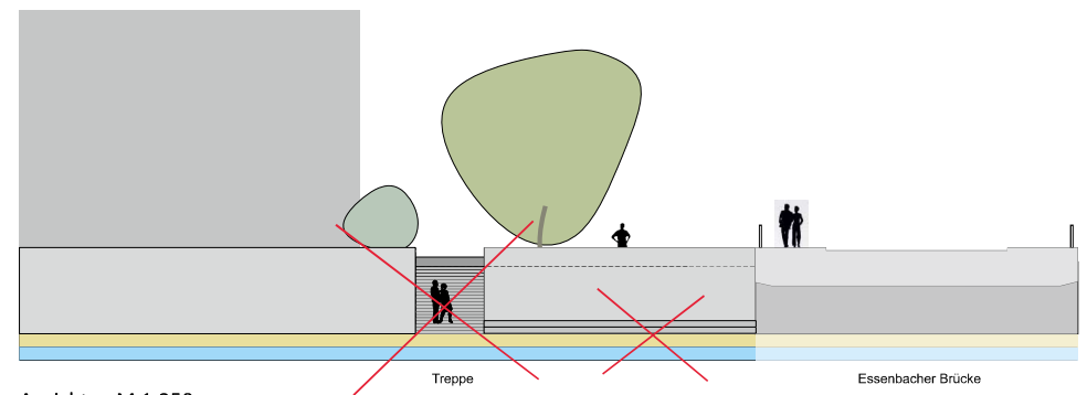
Ansicht M 1:250
