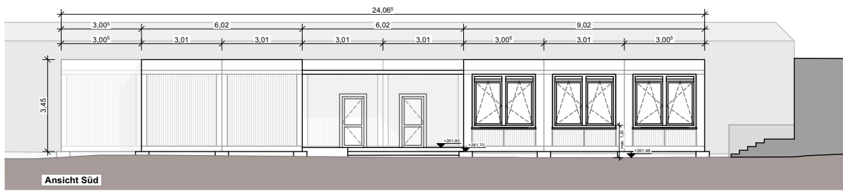
Ansicht Süd
