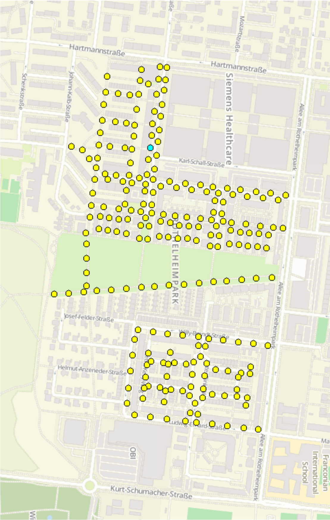
Anlage 1: Geplante Leuchtenstandorte für die Umrüstung
