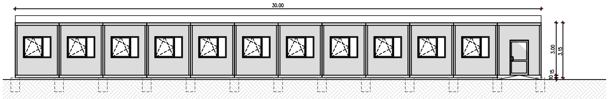
ANSICHT OST
