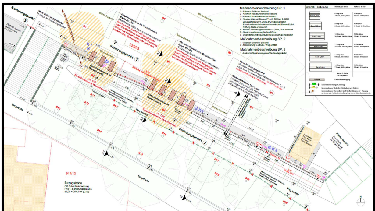
Anlage 4: Geländer-Sanierung im südlichen Bereich
