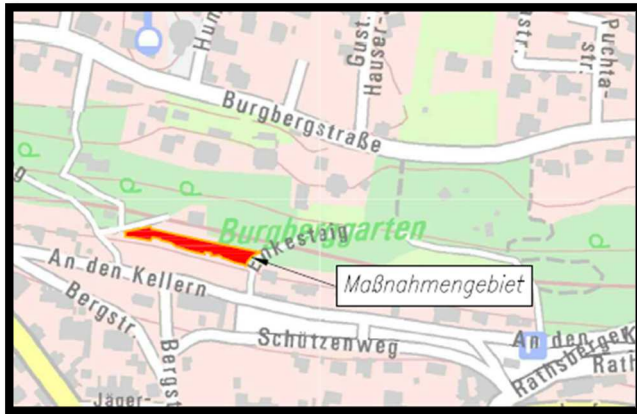
Anlage 3: Sanierung der Sandsteinmauer im Bereich der Anwesen „An den Kellern 19“ und „Burgbergstr. 73“ oberhalb des oberen Flucht- und Rettungsweges
