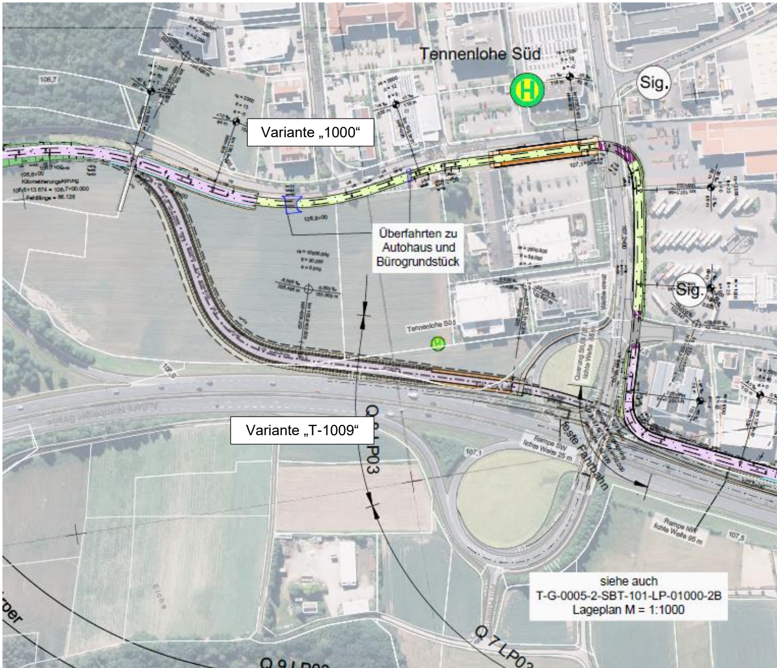
Anlage 1: Lageplan Varianten Wetterkreuz, Auszug aus Vorplanung T-G-0005-2-SBT-003-LP-02500-2B, Stand 23.09.2020
