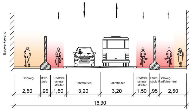
Straßenquerschnitt Unterführung Güterhallenstraße
