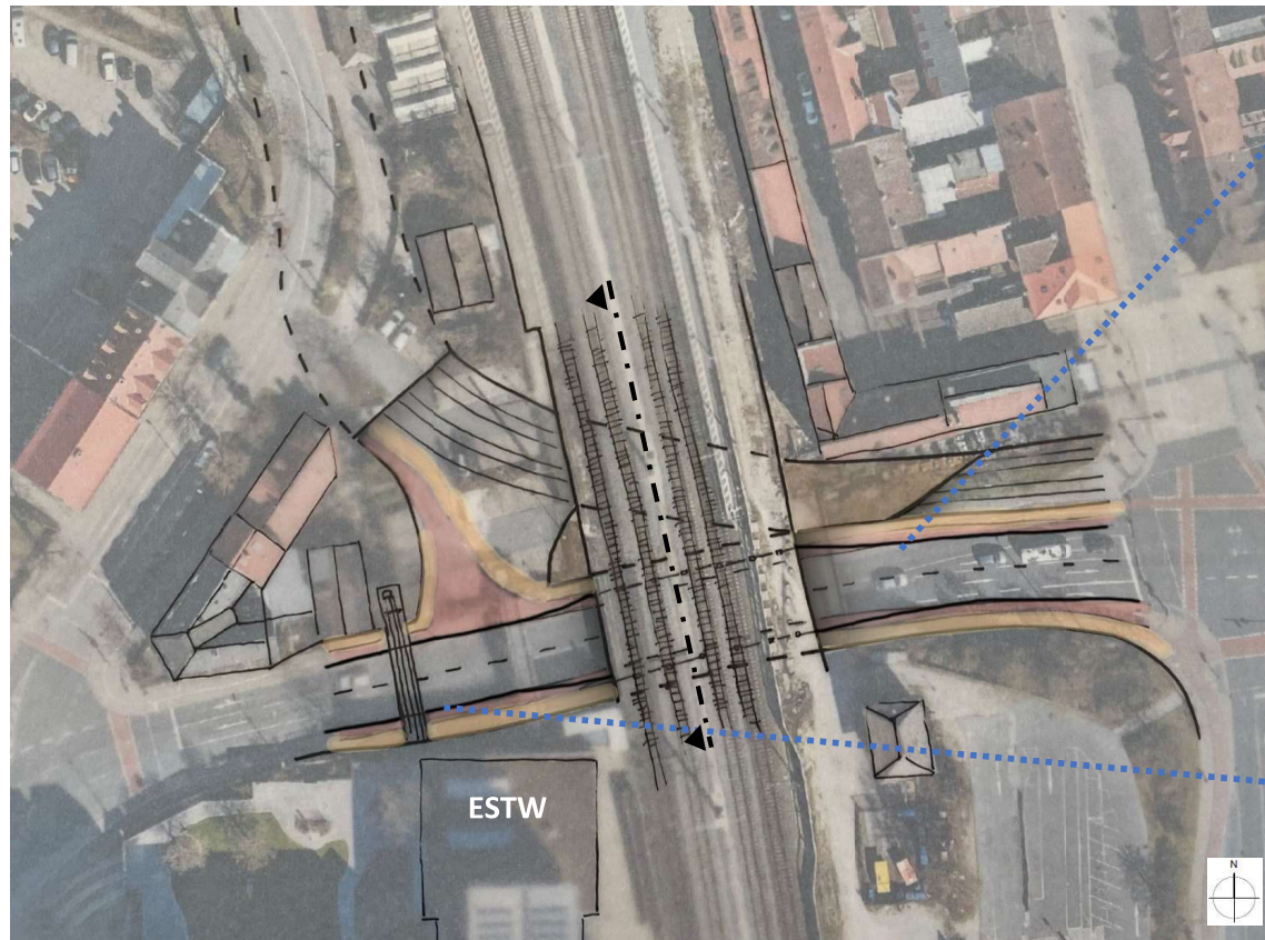
Lageplan Unterführung Güterhallenstraße
