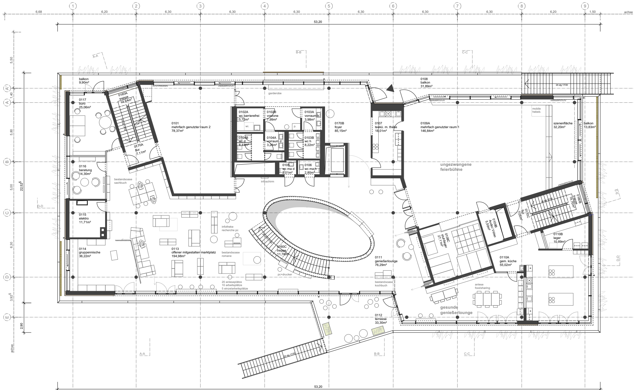
Entwurf 11.04.2022 0 1 2 5 10 m Stadteilzentrum mit Stadteilbibliothek Büchenbach
