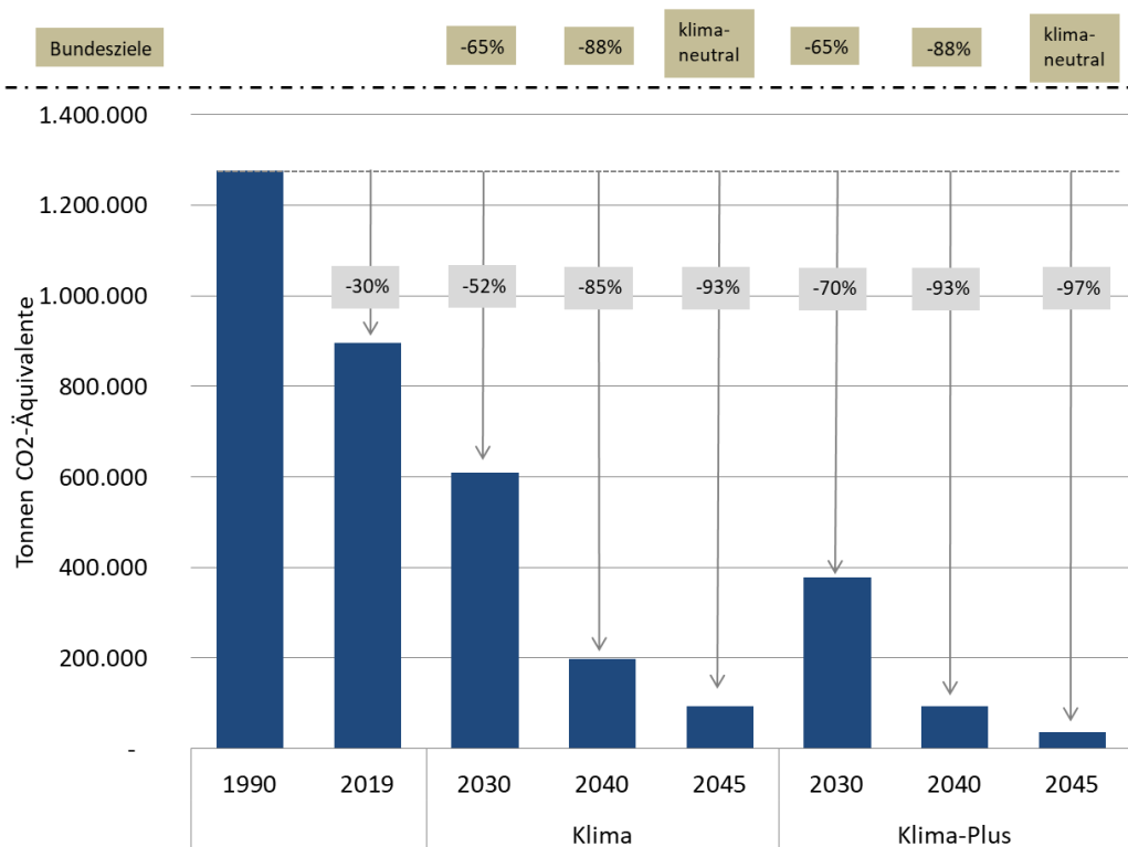
Abbildung 3-21: THG-Emissionsreduktion der Szenarien im Vergleich zu den Bundeszielen
