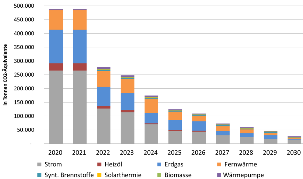
Abbildung 3-2: THG-Emissionen im 1,5-Grad-Szenario
