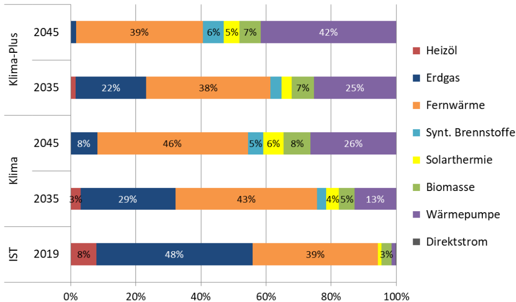
Abbildung 3-15: Entwicklung des Wärmebedarfs nach Energieträgern in den Szenarien
