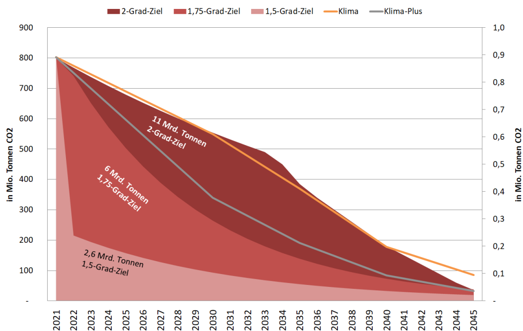
Abbildung 3-22: THG-Emissionen des Klima- und Klima-Plus-Szenarios in Relation mit dem CO 2 -Budget Deutschlands (angelehnt an Öko-Institut 2022)
