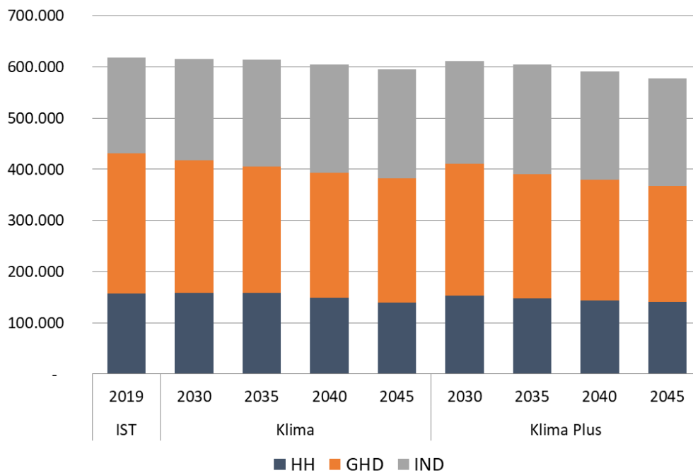
Abbildung 3-10: Stromverbrauch im Klima- und Klima-Plus-Szenario nach Sektoren
