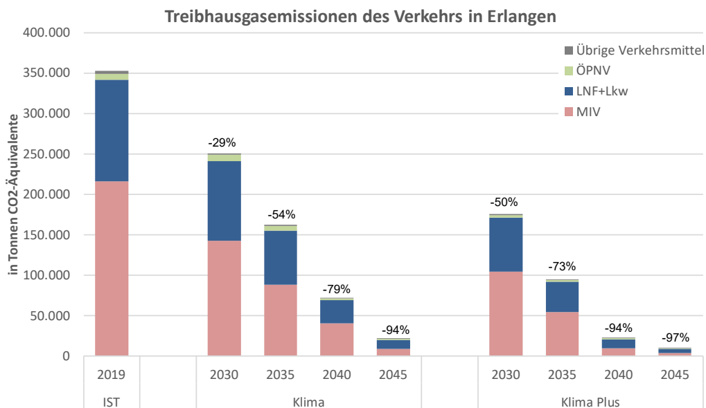
Abbildung 3-20: Entwicklung der THG-Emissionen im Verkehr im Klima- und Klima-Plus-Szenario
