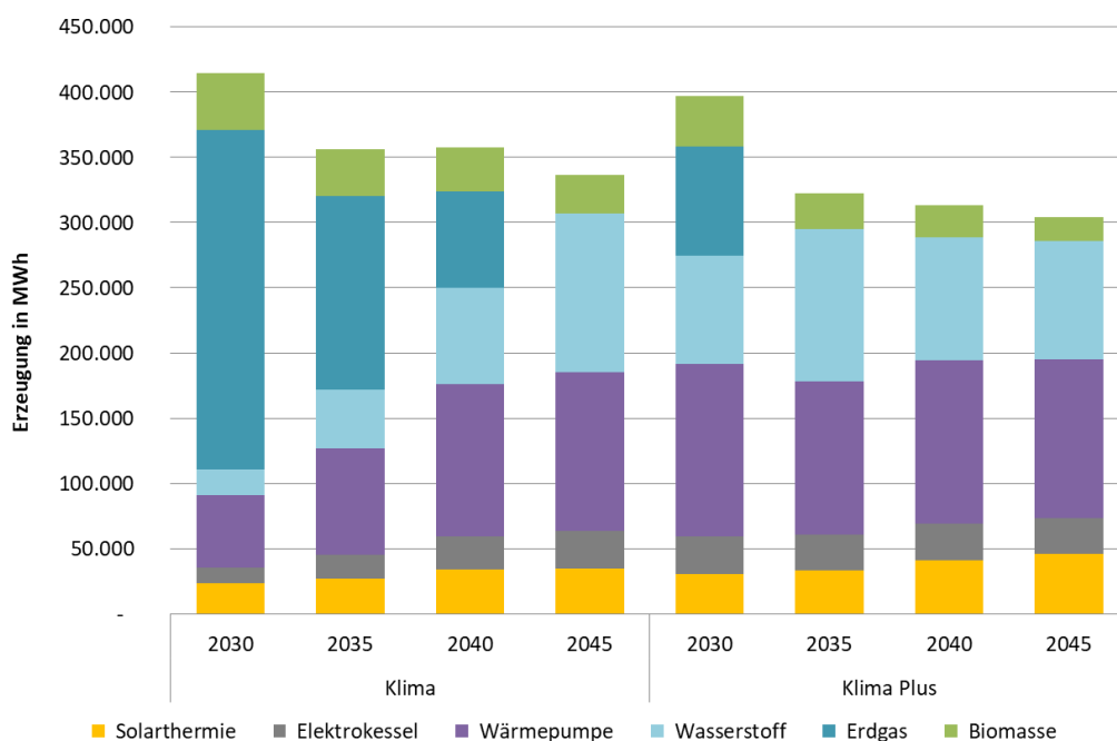
Abbildung 3-8: Fernwärmeerzeugung im Klima- und Klima-Plus-Szenario
