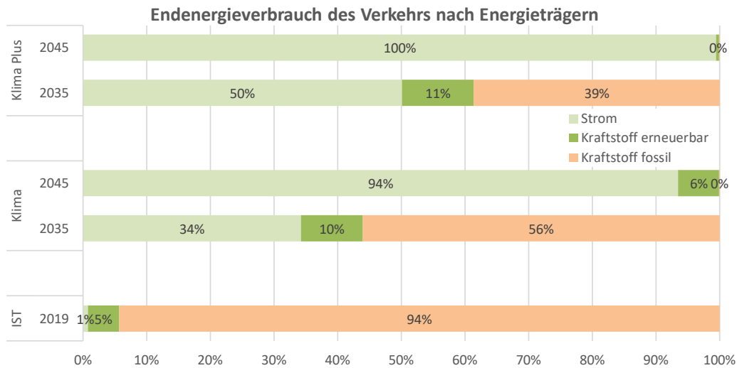
Abbildung 3-17: Endenergieverbrauch des Verkehr im Klima- und Klima-Plus-Szenario nach Energieträgern
