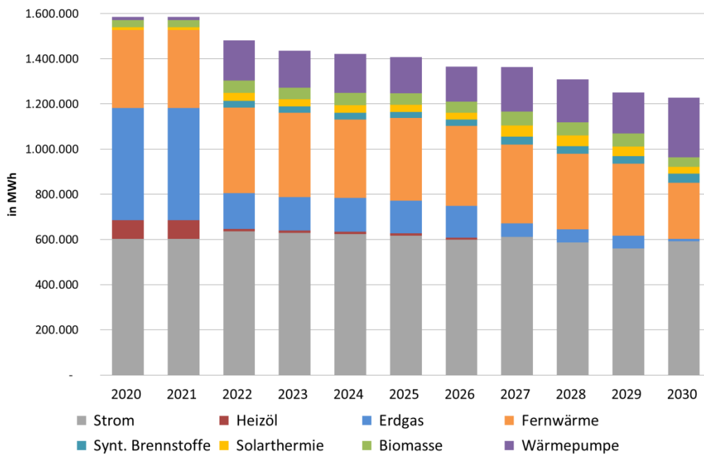
Abbildung 3-1: Energieverbrauch im 1,5-Grad-Szenario für den stationären Bereich nach Energieträger 1
