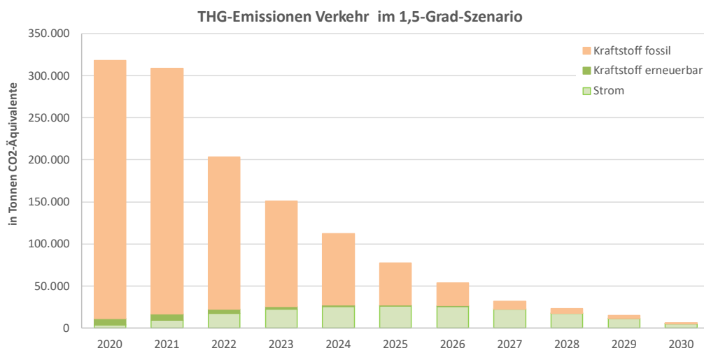
Abbildung 1-2: THG-Emissionen 1,5-Grad-Szenario im Verkehr
