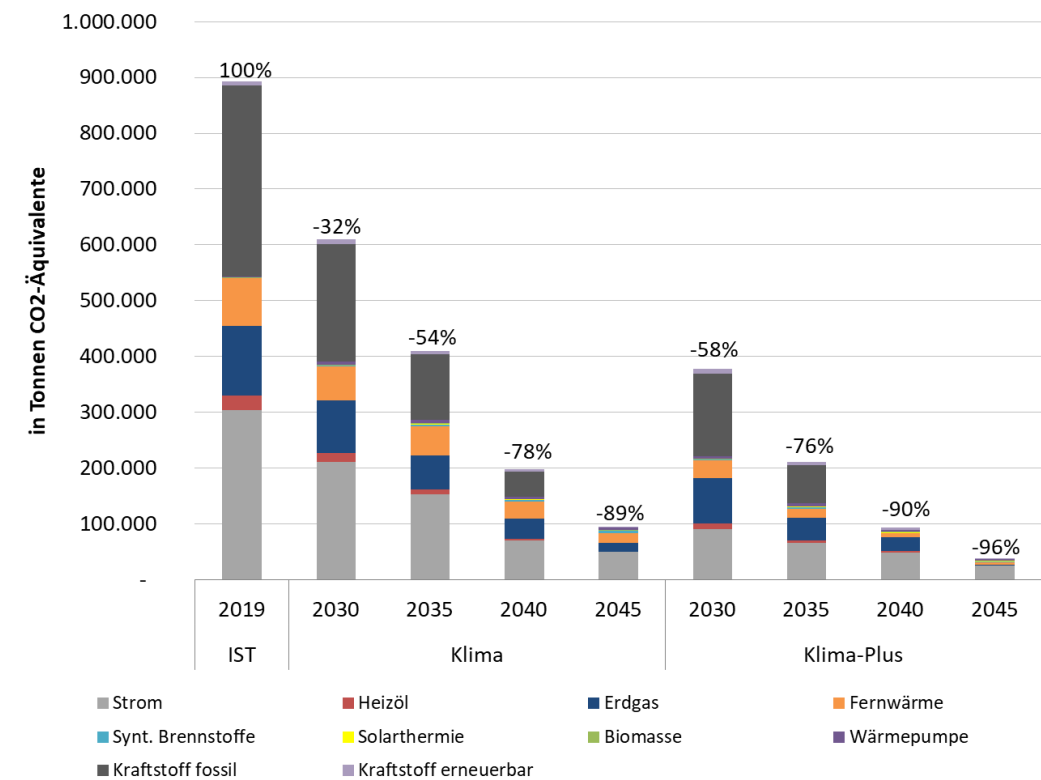
Abbildung 3-18: Entwicklung der THG-Emissionen im Klima- und Klima-Plus-Szenario
