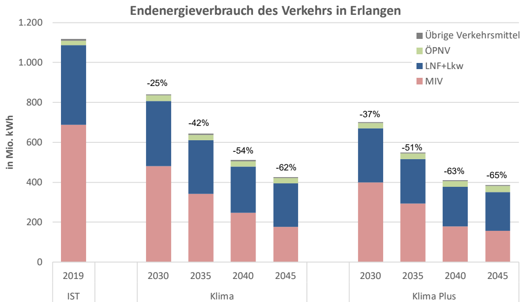
Abbildung 3-16: Entwicklung des Endenergieverbrauchs im Verkehr im Klima- und Klima-Plus-Szenario
