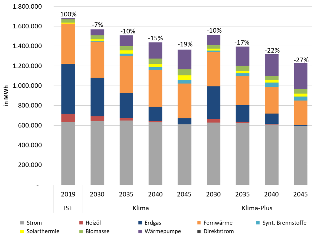
Abbildung 3-14: Entwicklung des stationären Endenergieverbrauchs im Klima- und Klima-Plus-Szenario
