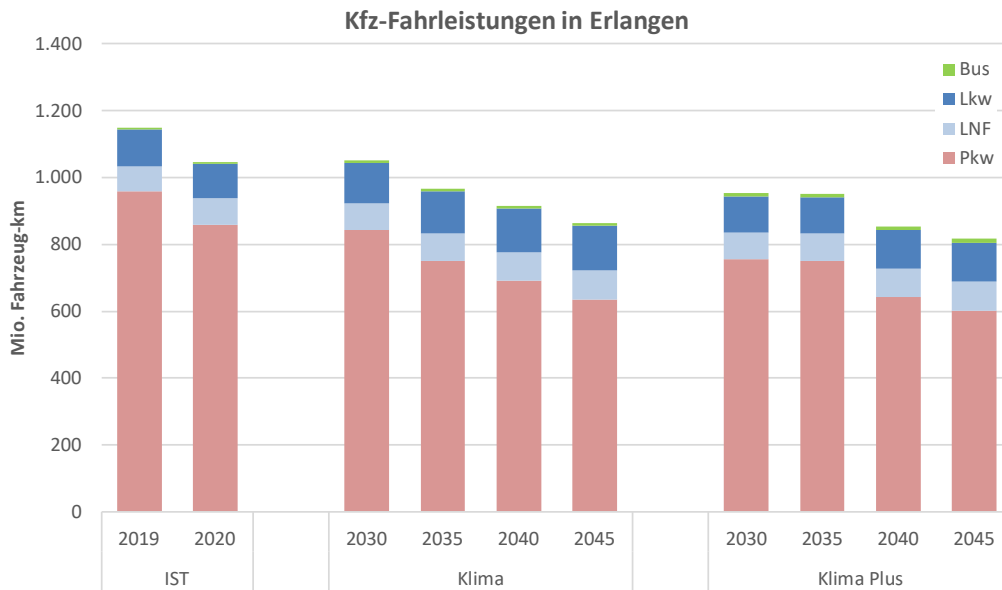
Abbildung 3-11: Fahrleistungen von Pkw (rot) und Lkw >3,5t (blau) in Erlangen
