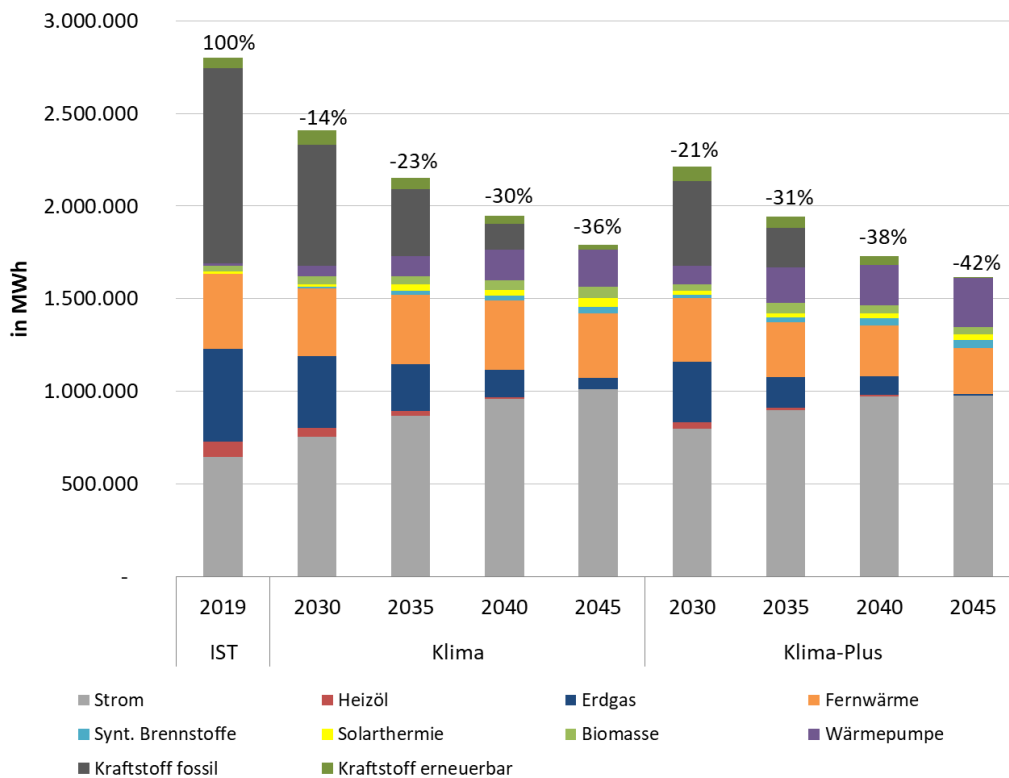
Abbildung 3-13: Entwicklung des Endenergieverbrauchs im Klima- und Klima-Plus-Szenario
