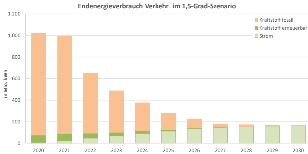
Abbildung 3-4: Endenergieverbrauch 1,5-Grad-Szenario im Verkehr
