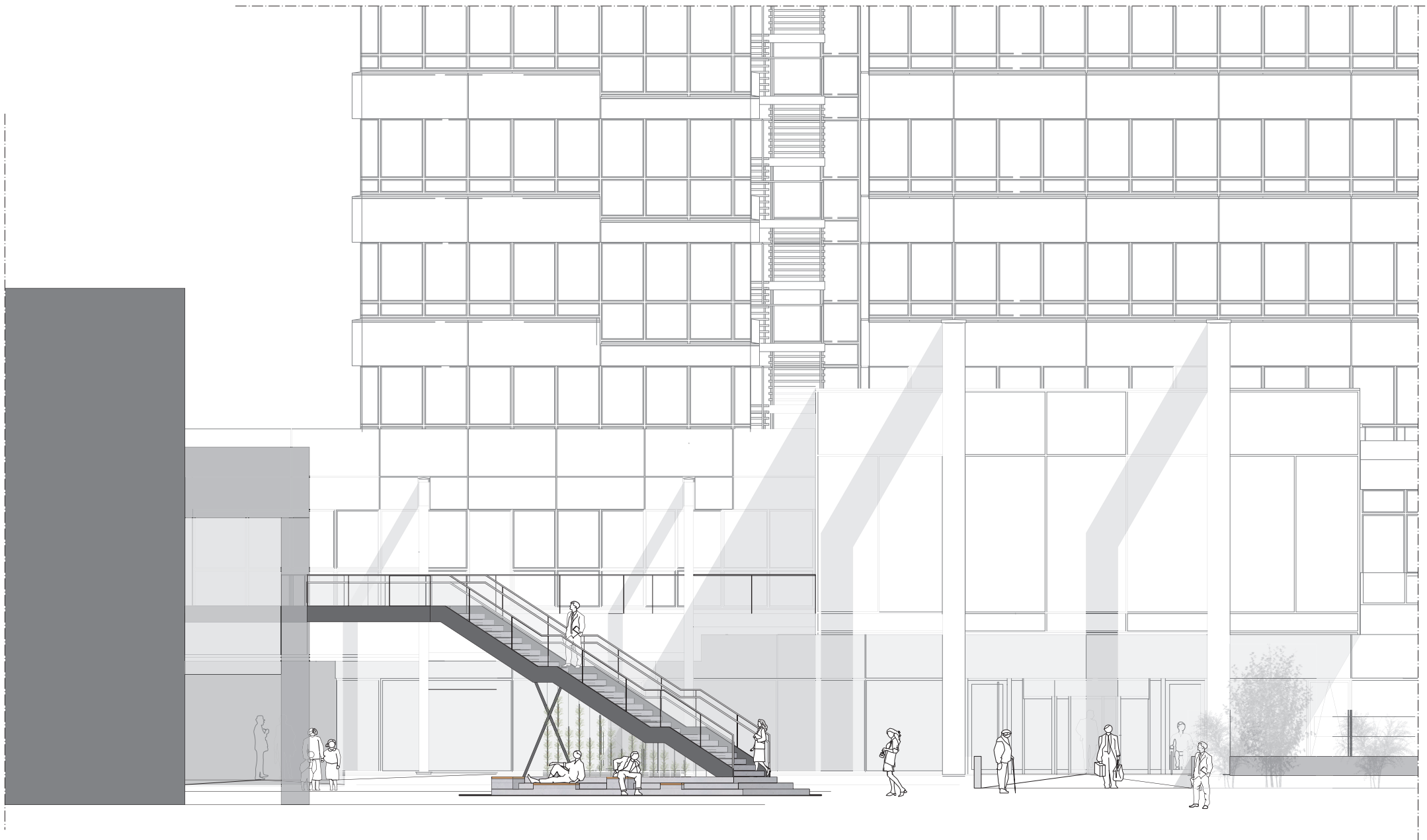
Neue Treppenanlage mittig zu Eingang Neuer Markt OG
