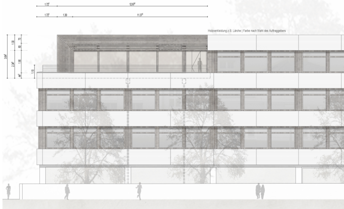
ANSICHT OST
