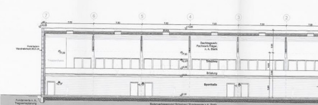
SCHNITT LÄNGS
