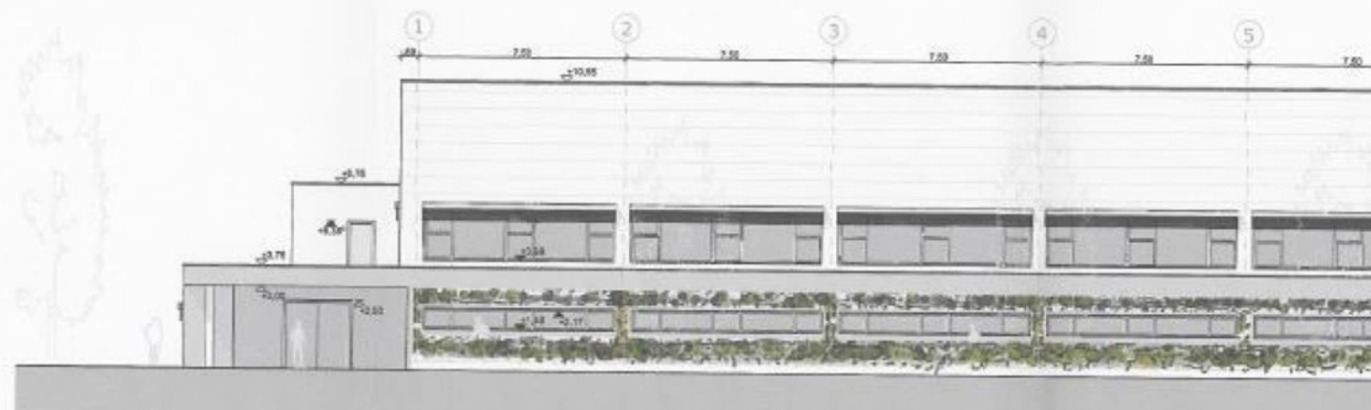
ANSICHT OST
