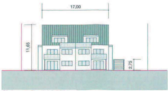
Schema-Ansicht-Süd
