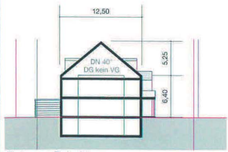
Schema-Schnitt
