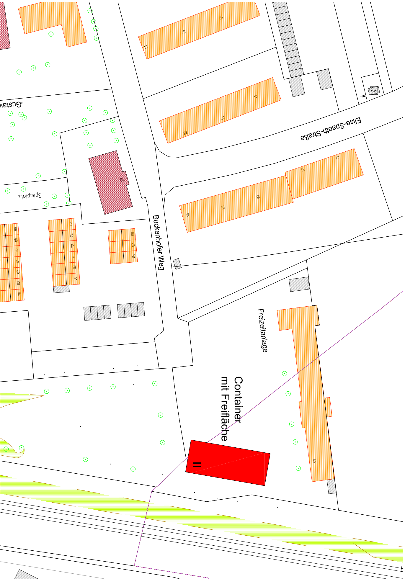
Standort einer temporären Kindertageseinrichtung Buckenhofer Weg/Brucker Radweg Übersichtsplan M. 1:1000
