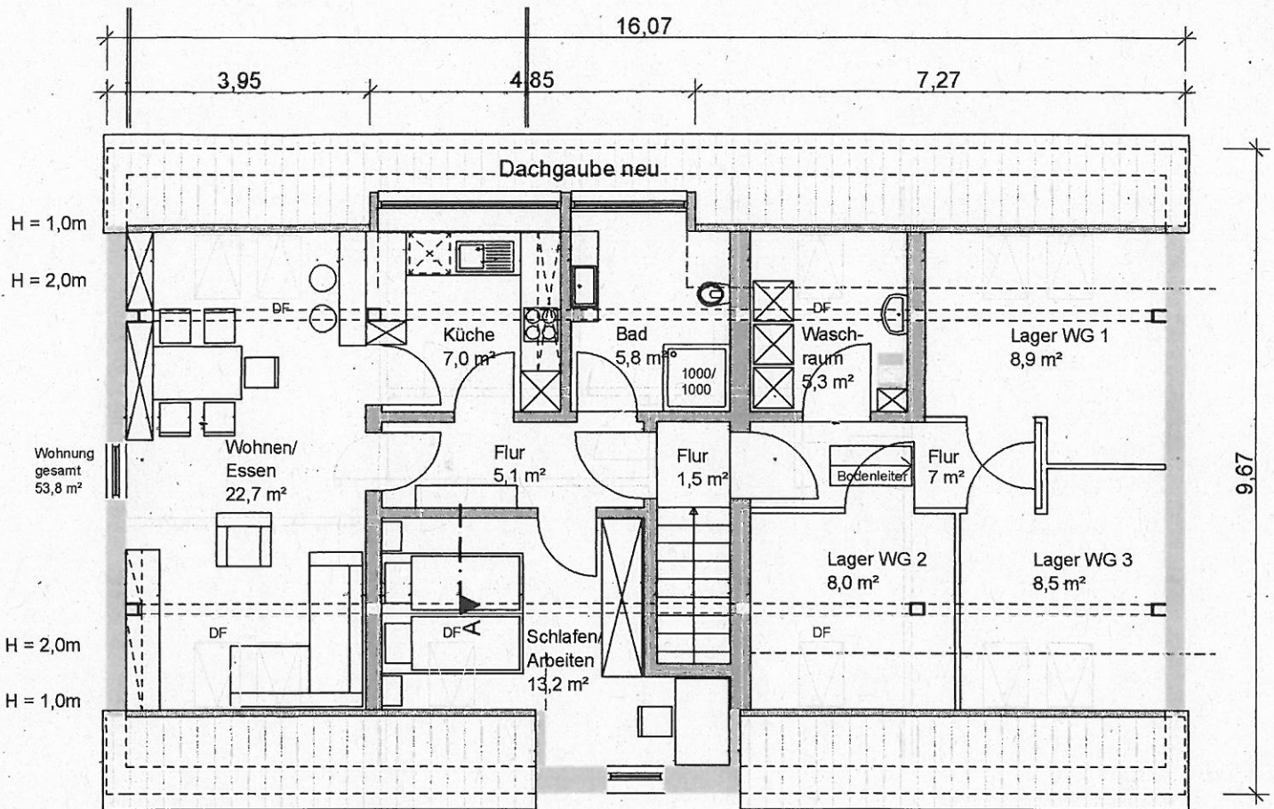
Dachgeschoss (Umbau)
