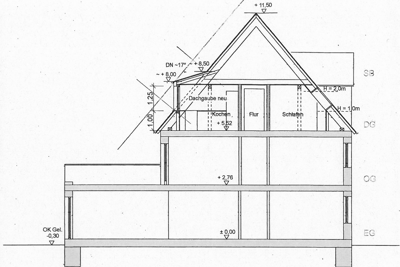
Schnitt A-A
