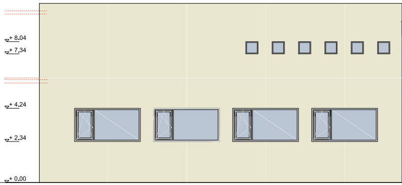
ANSICHT von NORDEN 1:100
