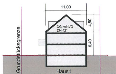
Schemaschnitt B-B
