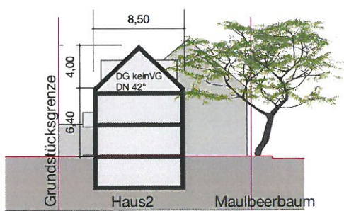
Schemaschnitt A-A
