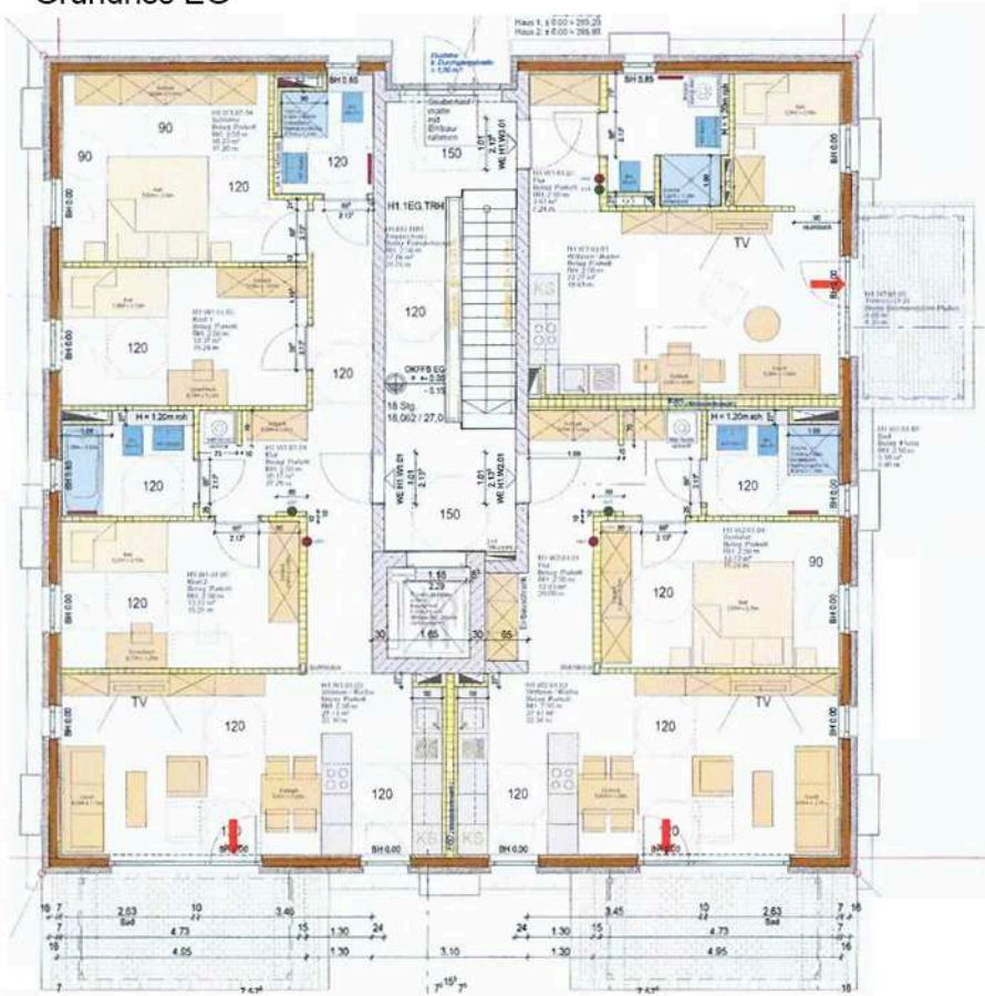
Grundriss EG
