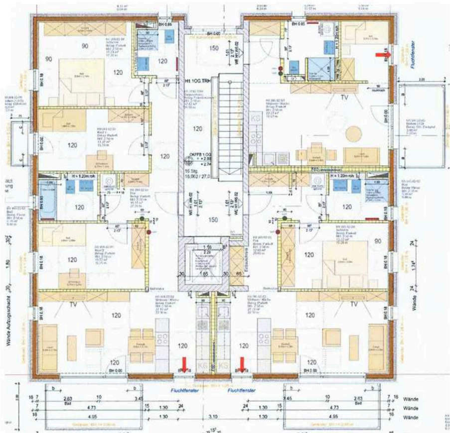
Grundriss 1. und 2. OG
