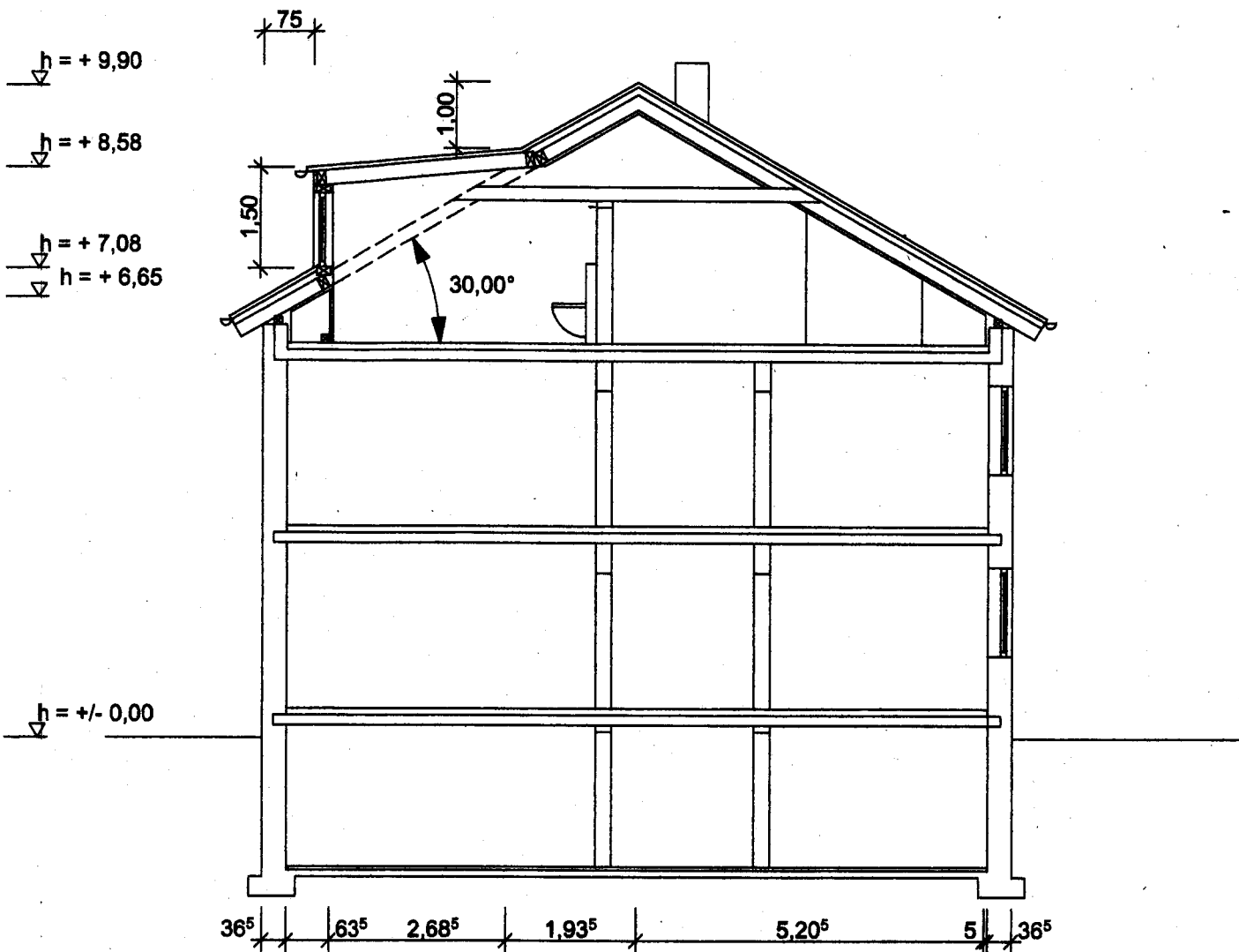
Schnitt M1:100
