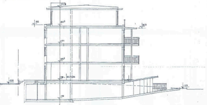
SCHNITT B B
