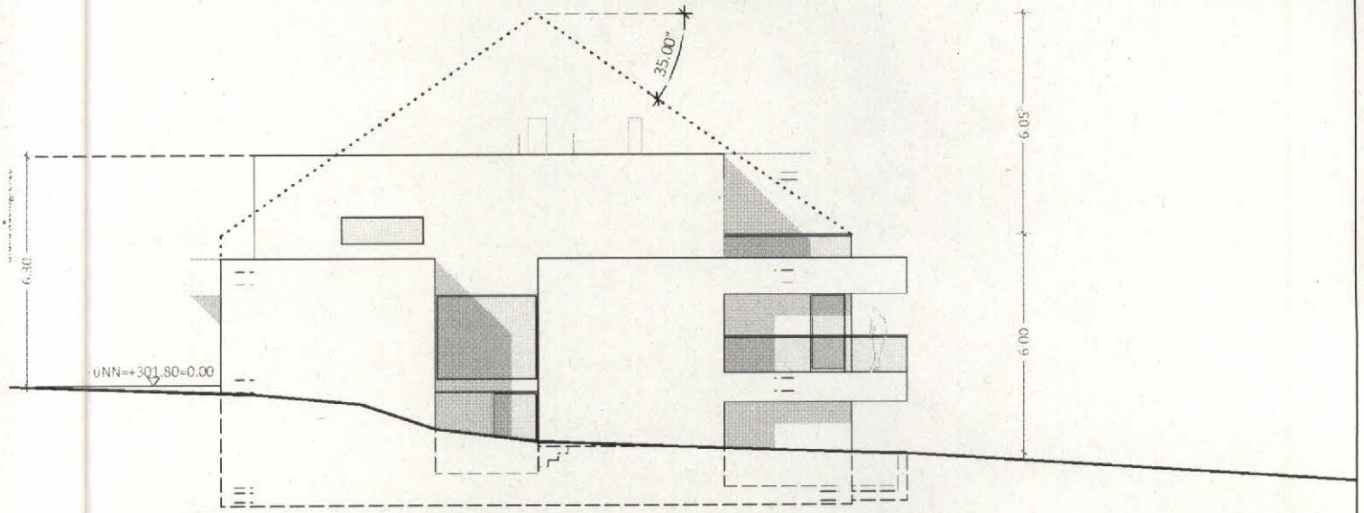
Ansicht Ost
