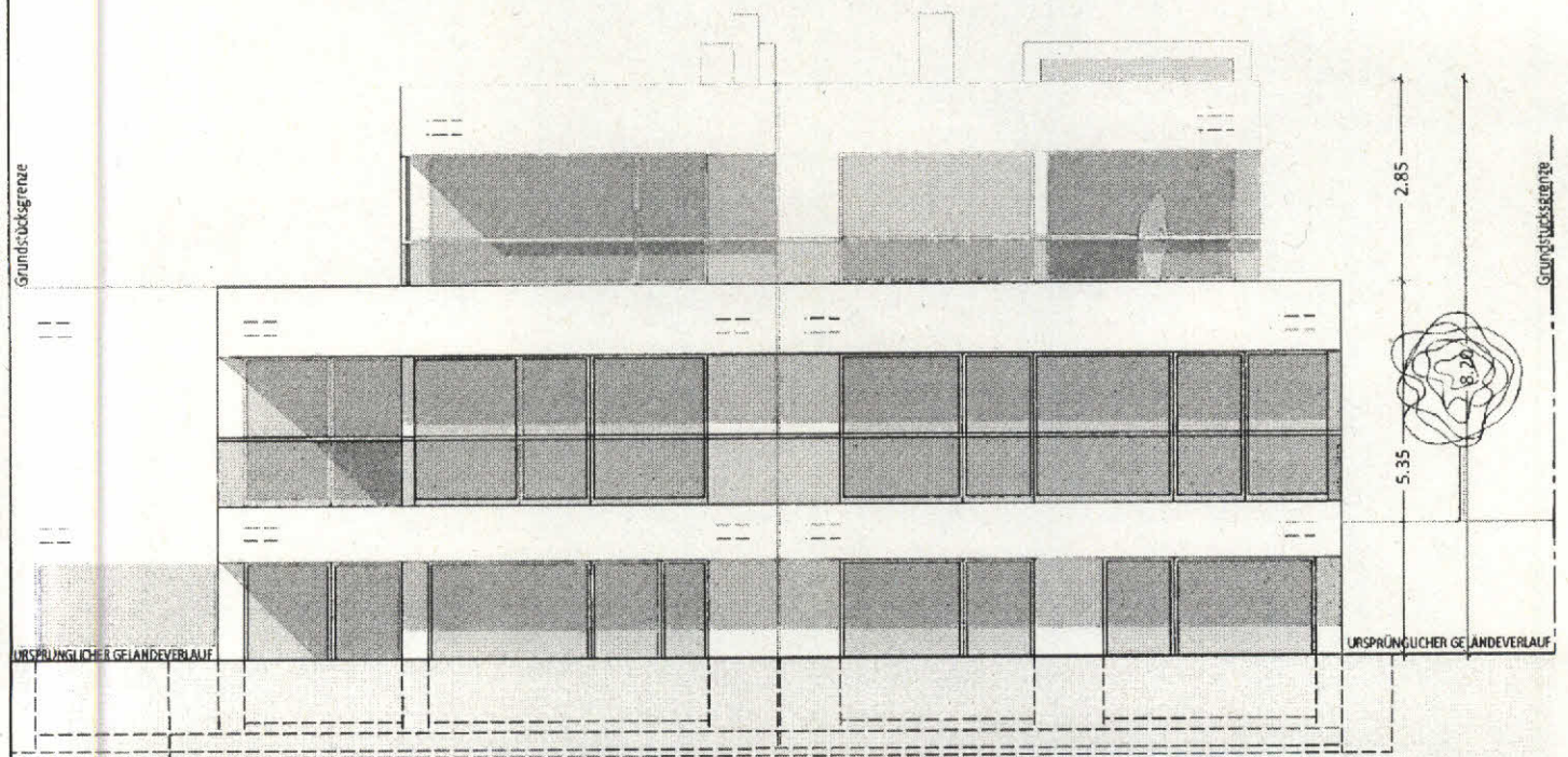
Ansicht Süd
