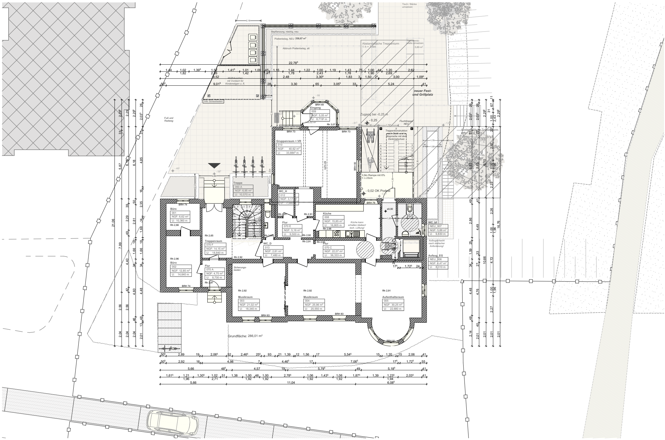
ERBA Villa | Wiedernutzbarmachung OG + DG + barrierefreie Erschließung | Übersicht | M = 1 : 200
