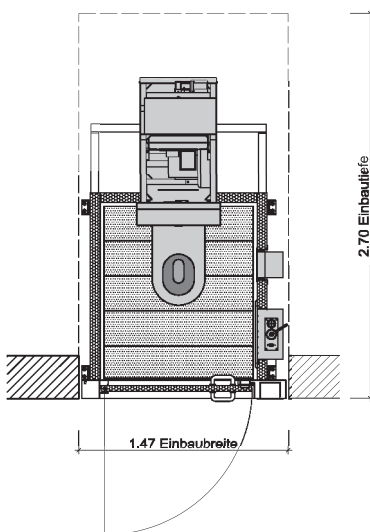
Einbaumaße: FLEXI KIT Mini mit SBR
