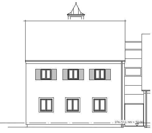
Ansicht Ost
