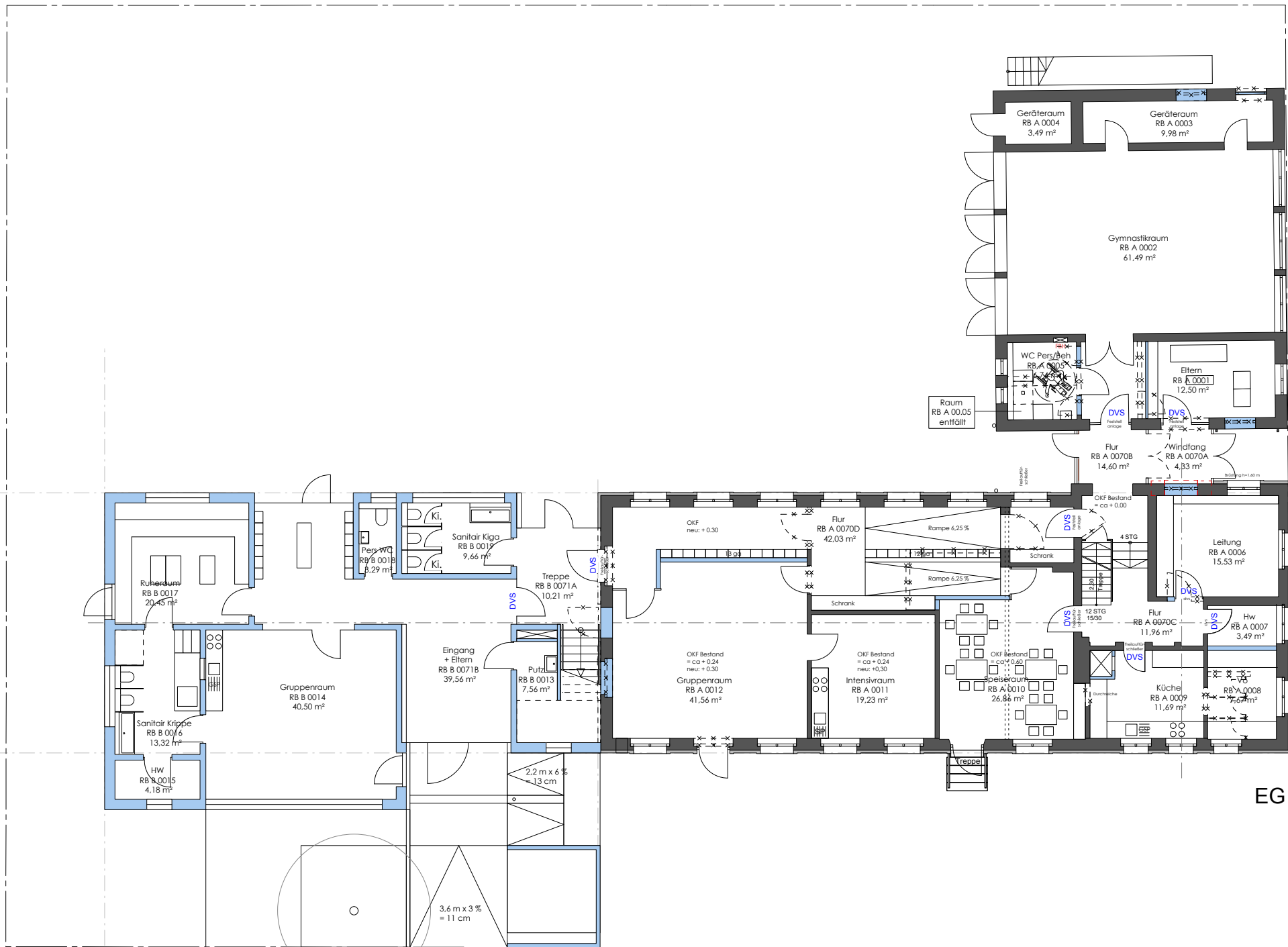
Anbau Kinderkrippe mit Umbau und Sanierung Kindertageseinrichtung 'Flohkiste', Hans-Sachs-Straße 2, 91056 Erlangen Vorentwurf 24.09.12, Rößner + Waldmann
