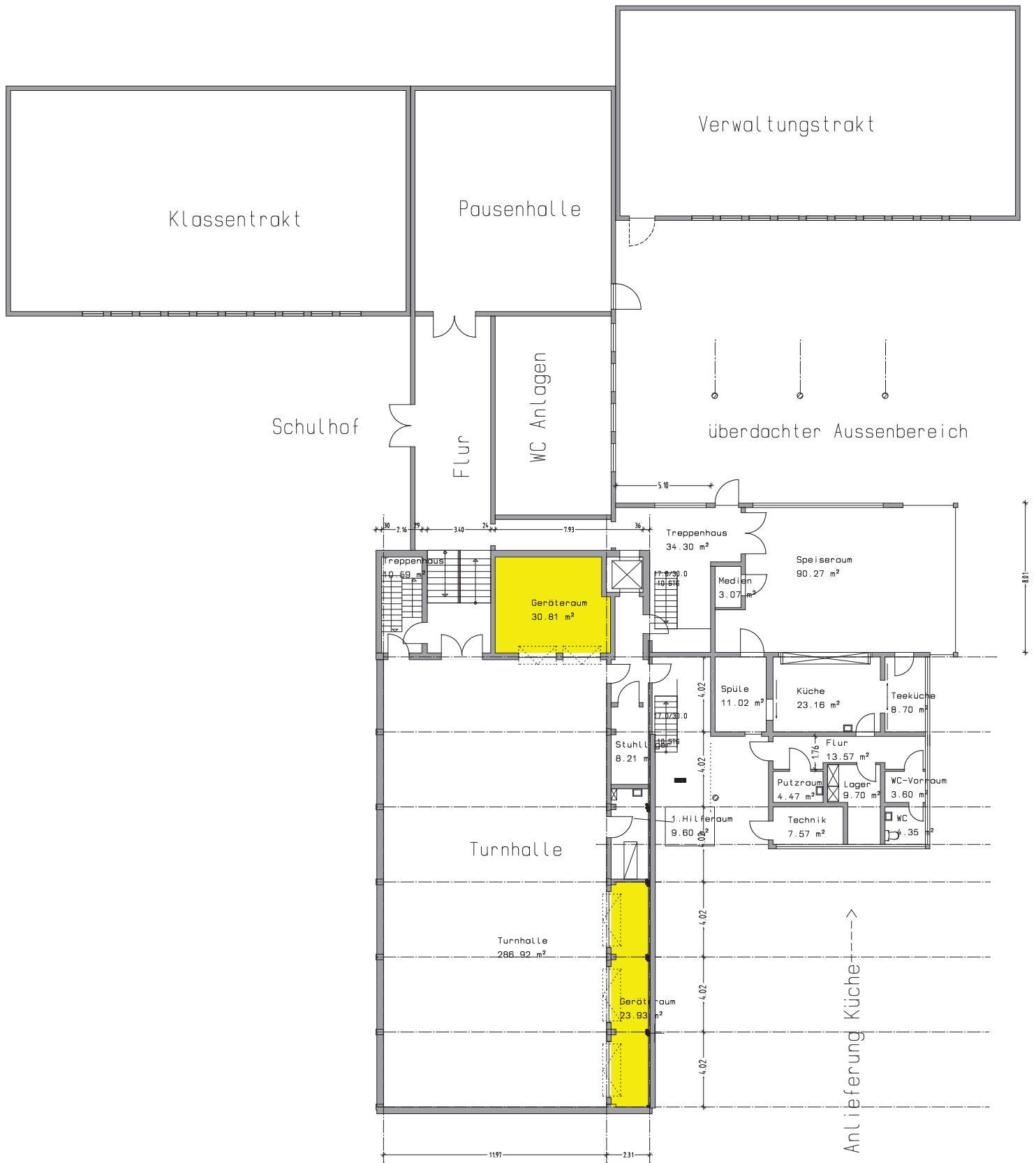
Ganztagesbetreuung Tennenlohe mit Turnhalle EG
