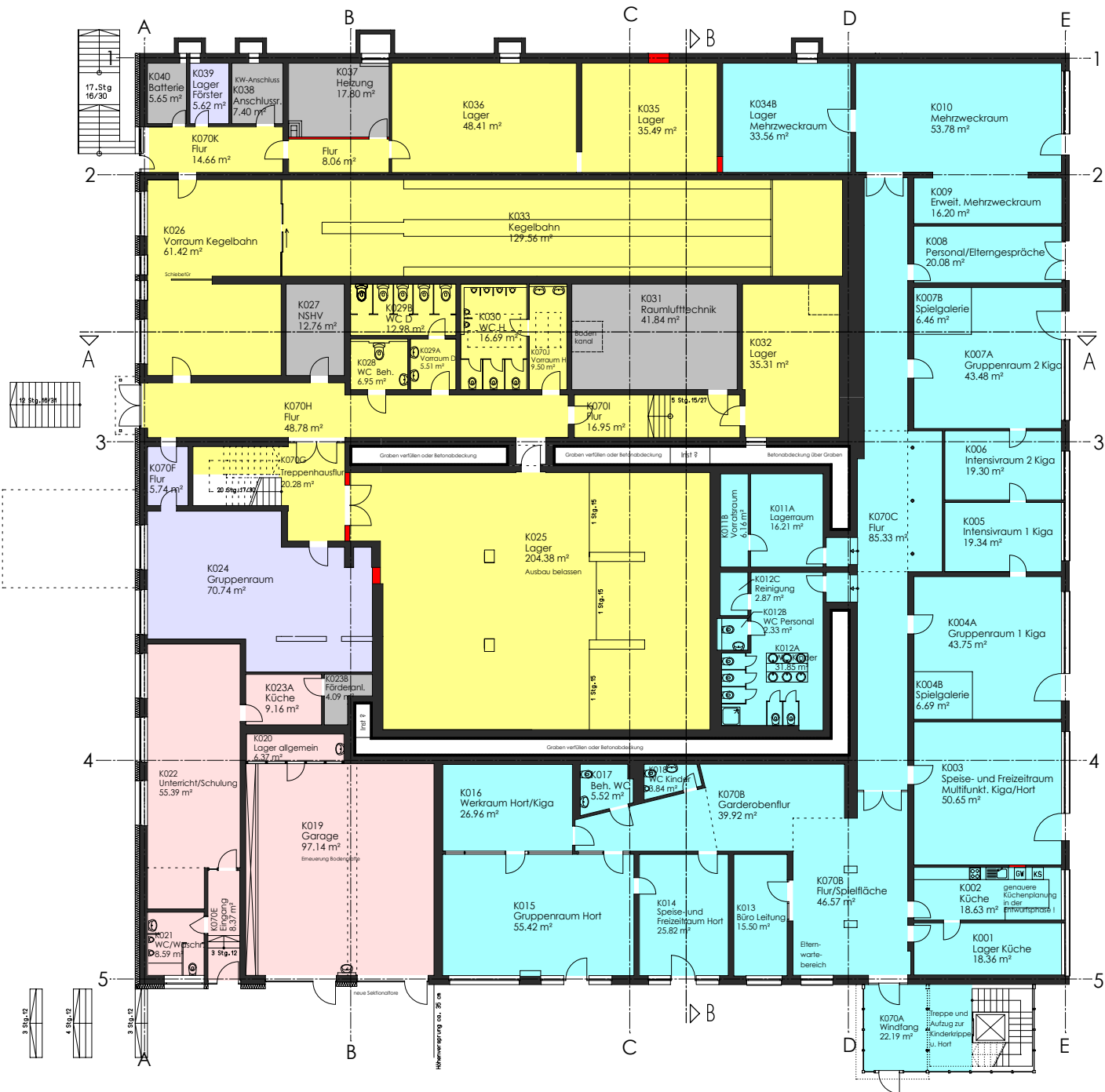
Gemeindezentrum Frauenaurach - Kellergeschoss - Variante 2
