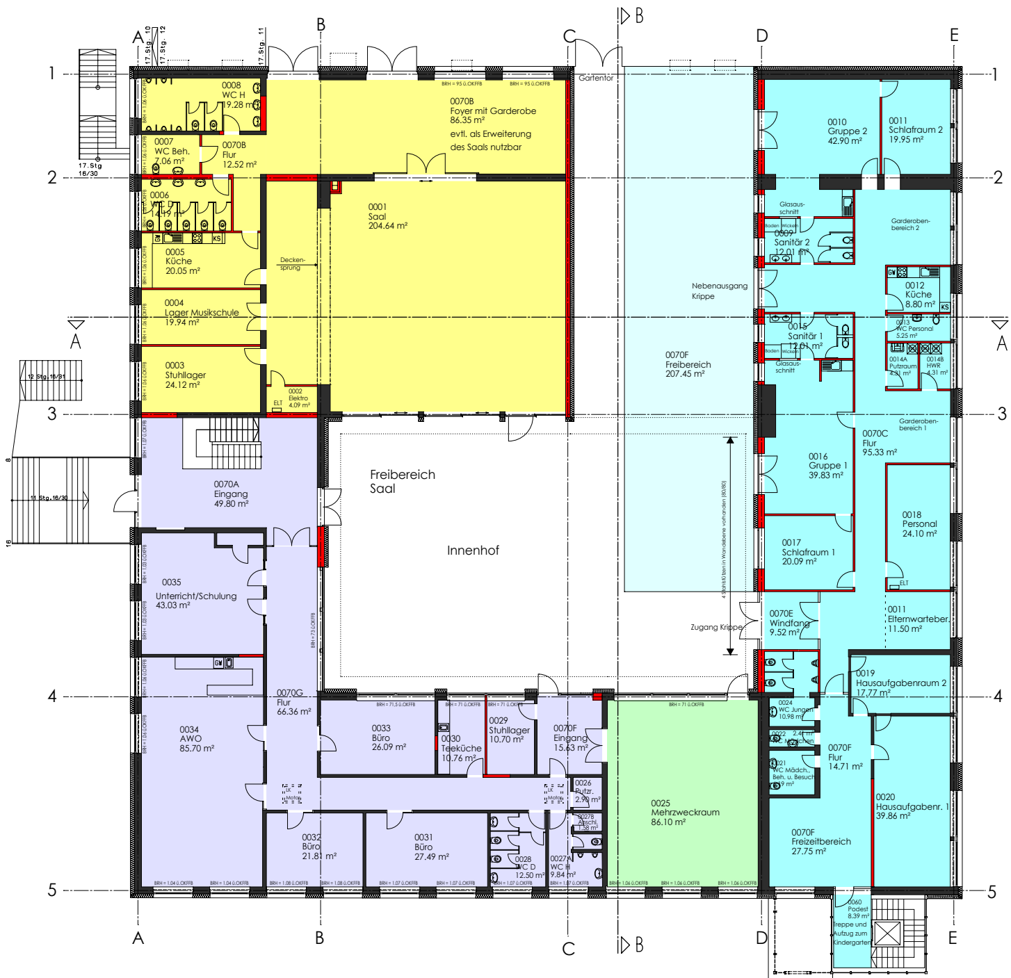
Gemeindeforum Frauenaurach - Erdgeschoss - Variante 1
